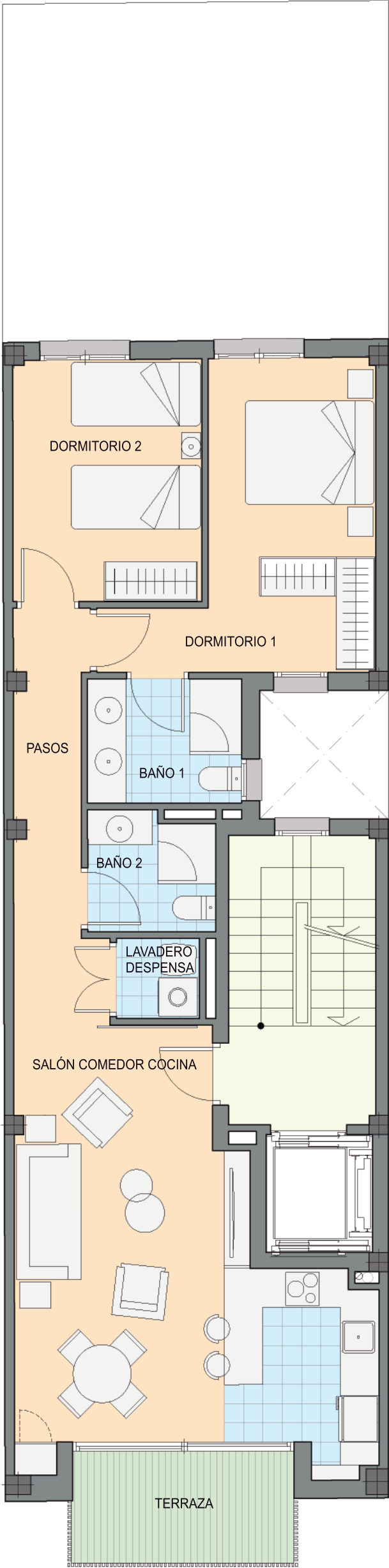
PLANTA 2ª
