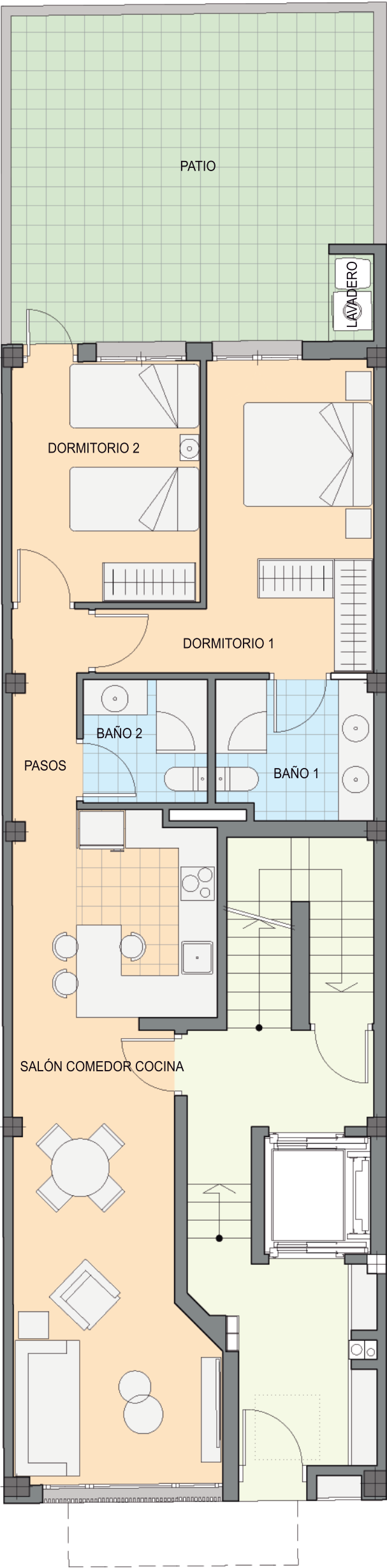
PLANTA BAJA
